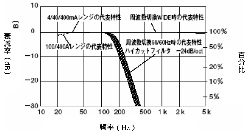
图3 M-2432、M-2433 频率特性
